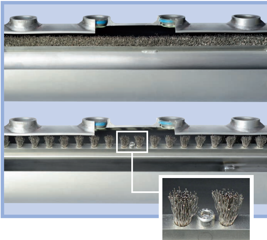
Bürste für kleine Rohre
